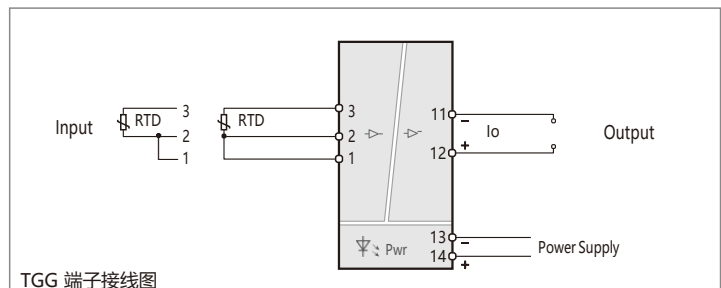
TGG 端子接线图
