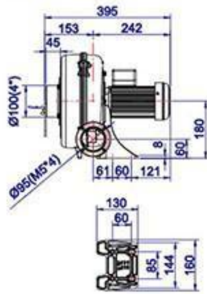
HTB75-032 2-stage
