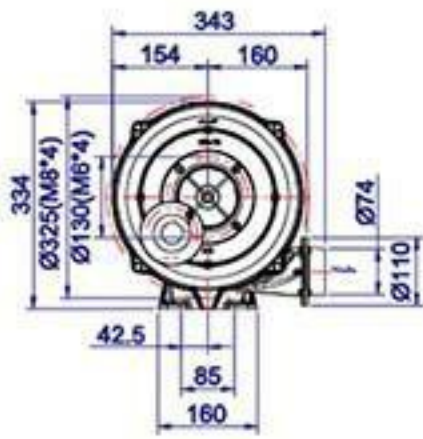
HTB75-032 2-stage
