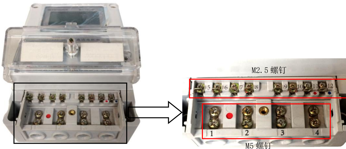
图 2 端子接线图
