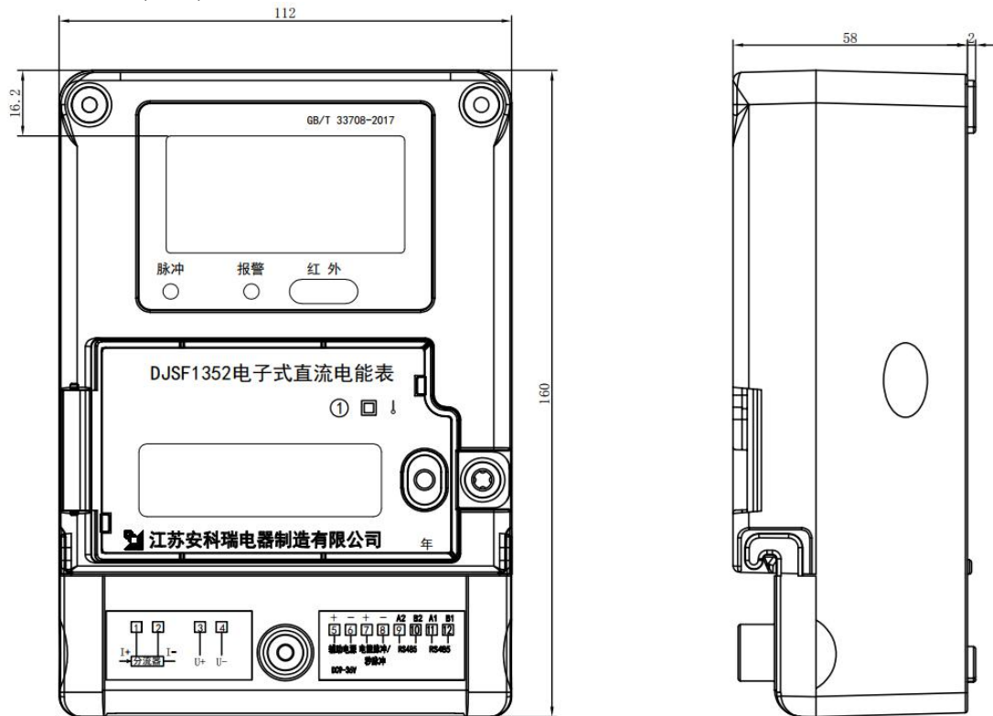
图 1 外观尺寸
