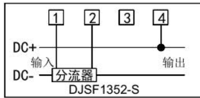
三线制共负接法
