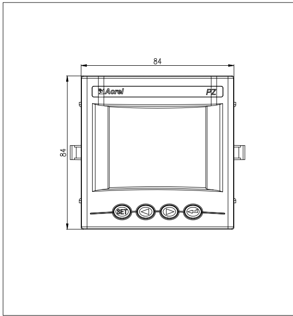
图 5 PZ80 安装尺寸
