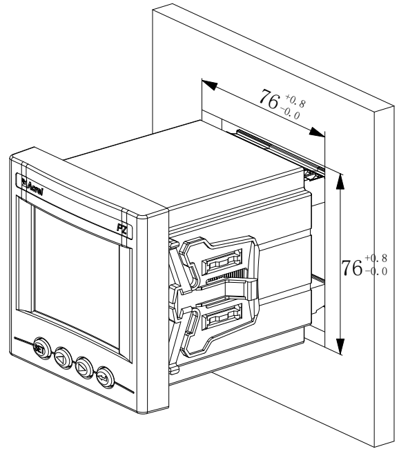
图 5 PZ80 安装尺寸
