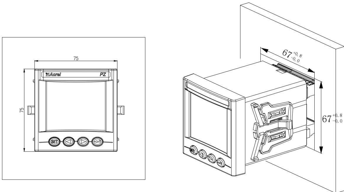
图 4 PZ72 安装尺寸
