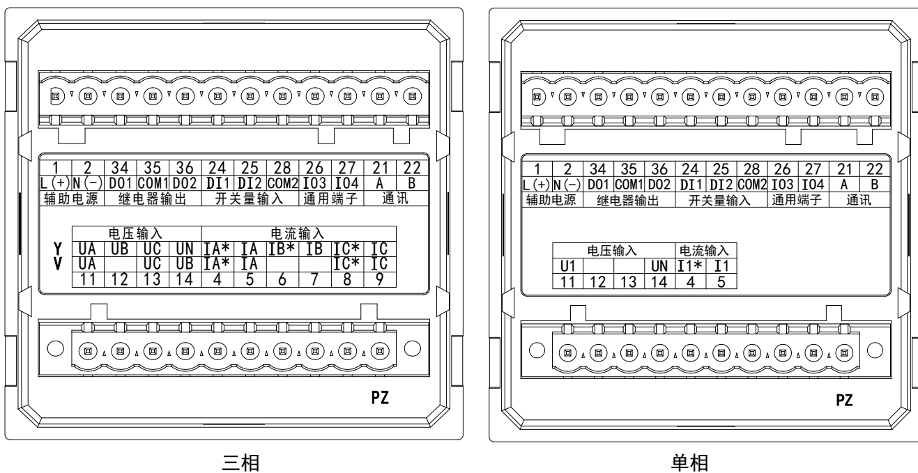
图 9 PZ72 系列接线端子图
