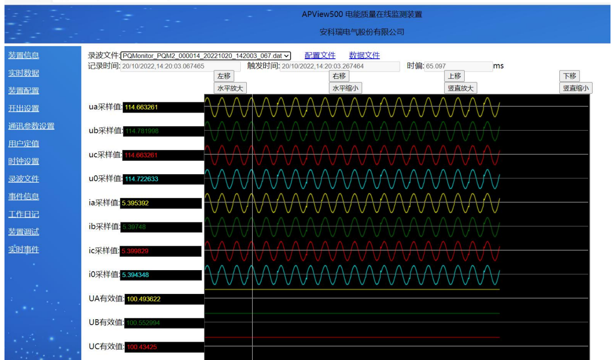
图 1.4 波形界面
