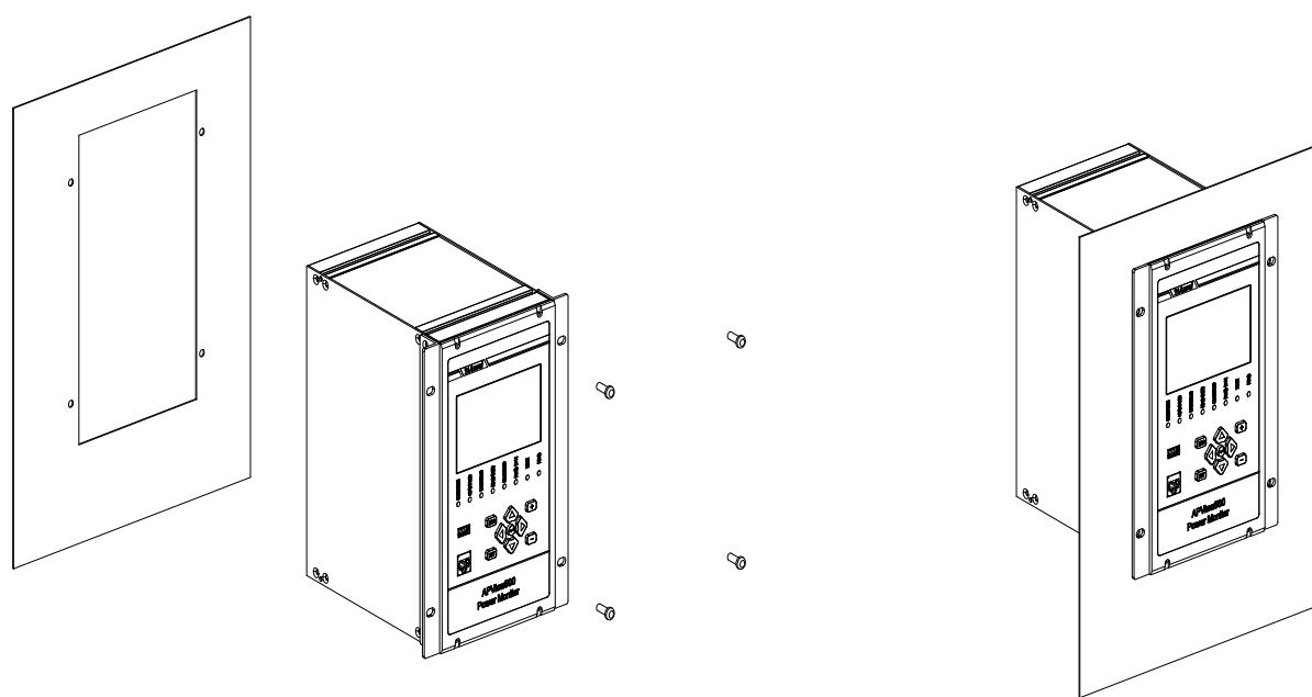
图 3.2 安装示意图
