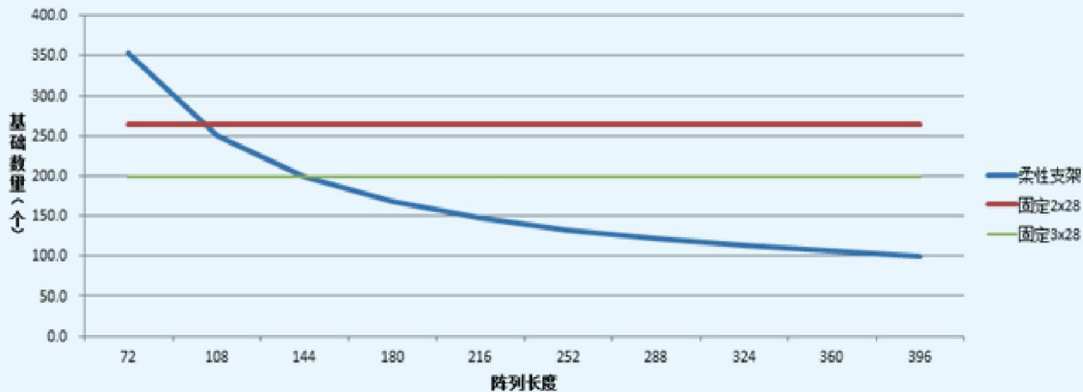
平地柔性与固定支架基础数量对比
