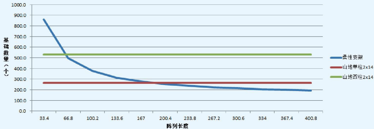
山地柔性与固定支架基础数量对比
